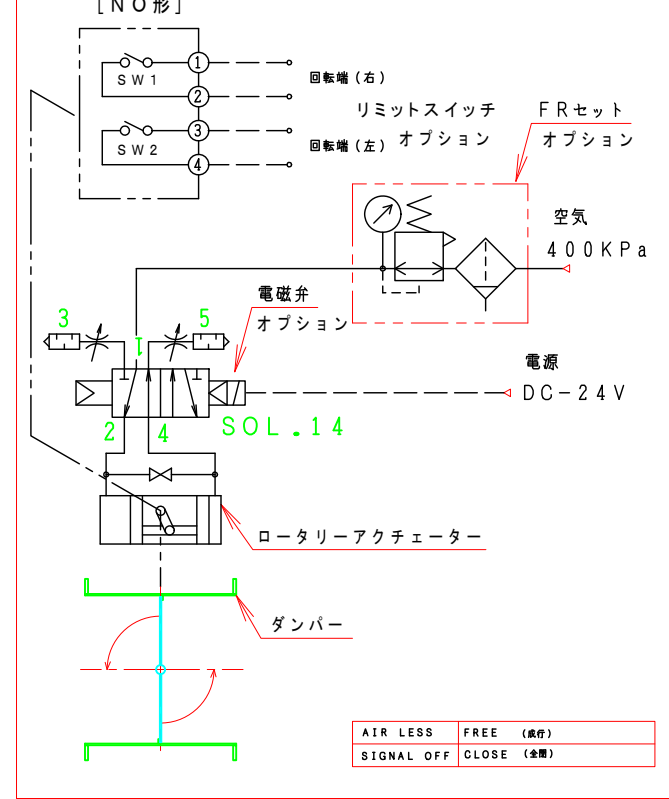
フローシート図 [TA2-063D-□□-□□□]
